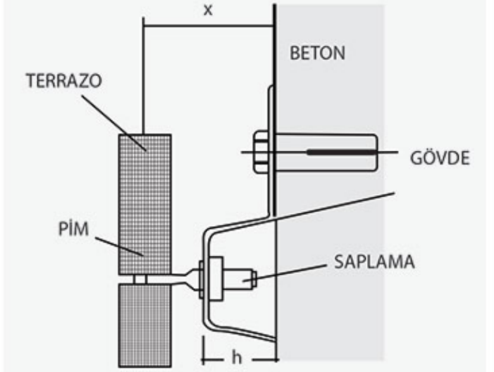
Teknik Çizim
