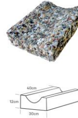
B-26 SU OLUĞU
