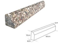
B-26 DÜZ BORDÜR 1
